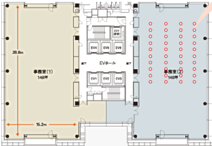
【平面図】
